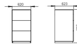
W1016 3-lådsmodul
